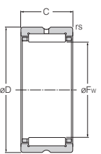
RNA49 -- R (øFw ≥ 14 mm) RNA59 RNA69 -- R NK -- R (øFw ≥ 14 mm)
